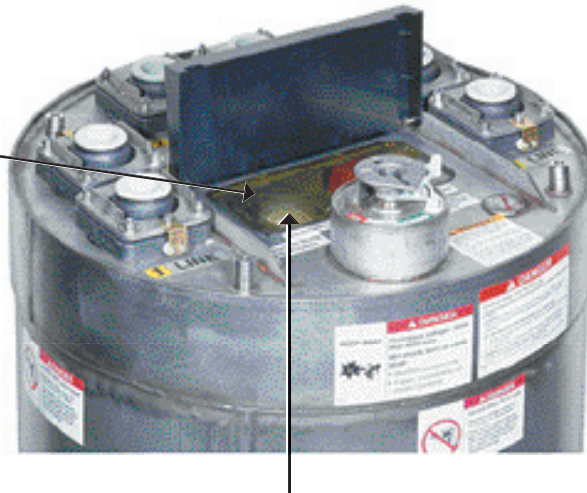
Medidor de presión (localizado debajo de la ventana) compensado por temperatura y altura.
